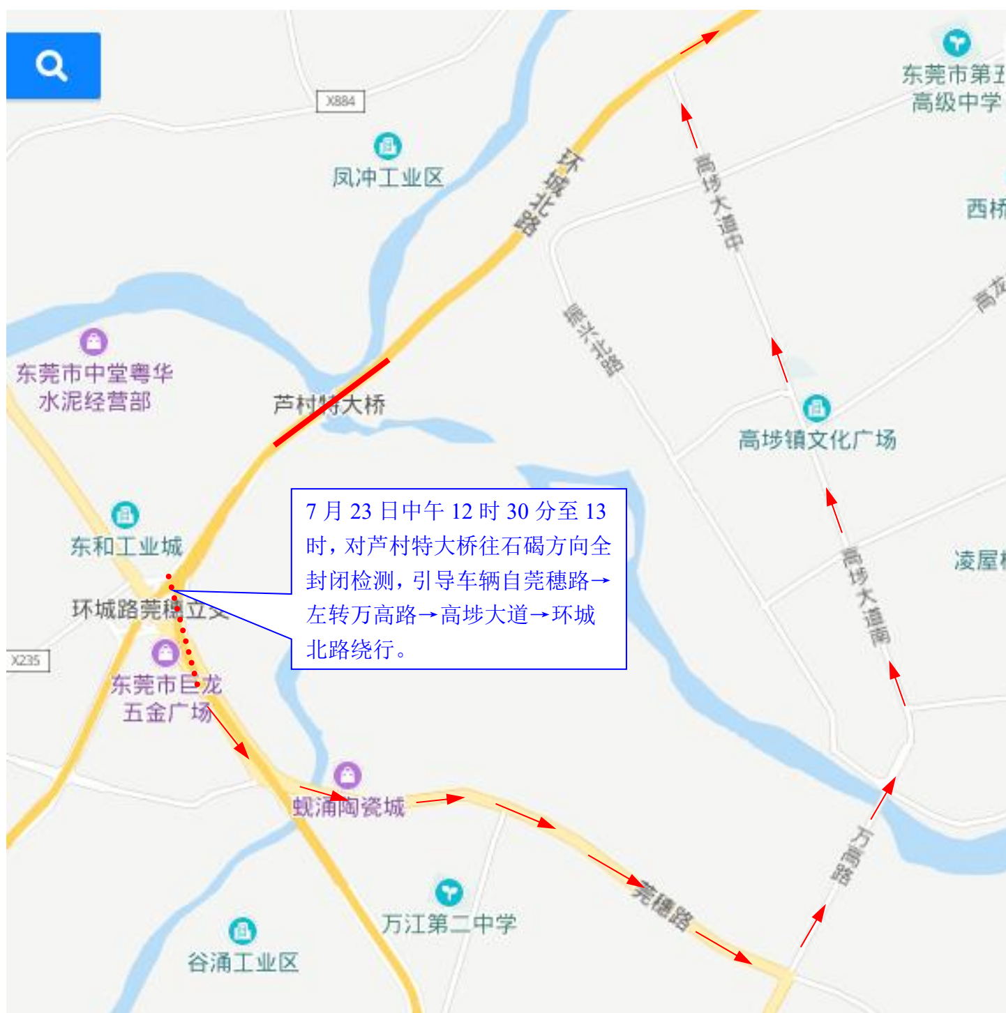
芦村特大桥主桥交通疏解图
